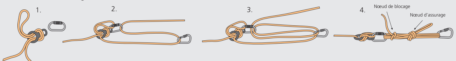
Détail d'un mouflage à l'aide d'un descendeur en huit
