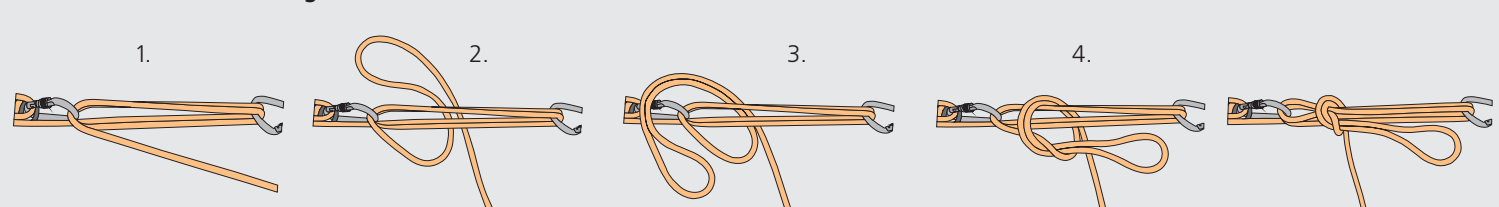
Détail du nœud de blocage
