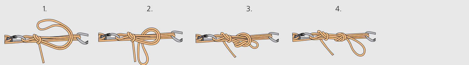
Détail du nœud d'assurage
